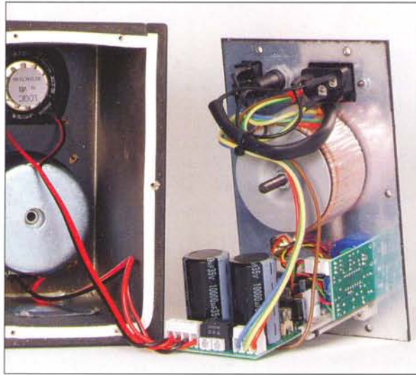
Pro Audio 30 on aktiivikaiutin pienoiskoossa. 55-mallissa on sama vahvistin, mutta hieman suurempi virtalähde.
